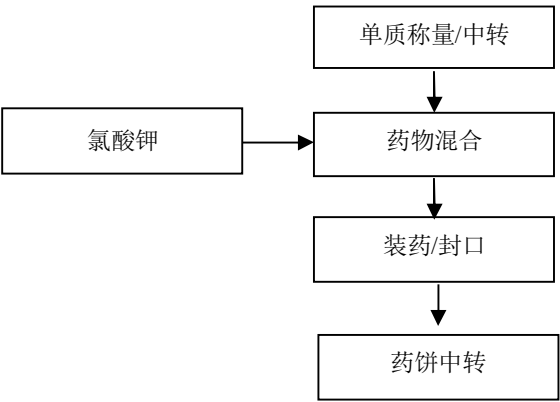
图 2-3：烟雾内筒生产工艺流程图
