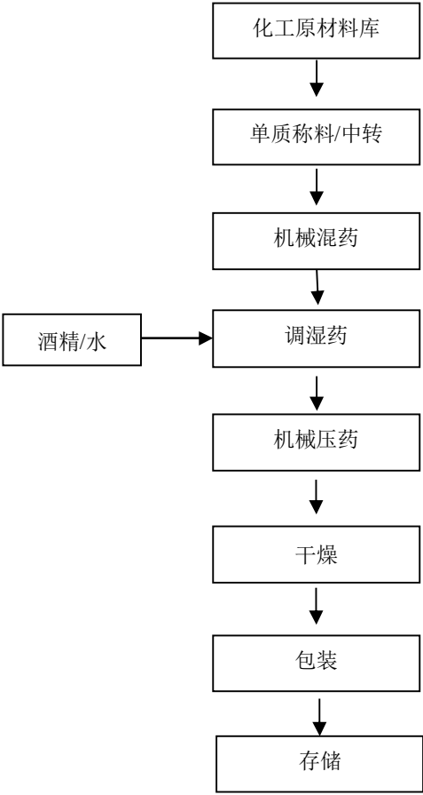
图 2-5：药柱生产工艺流程图
