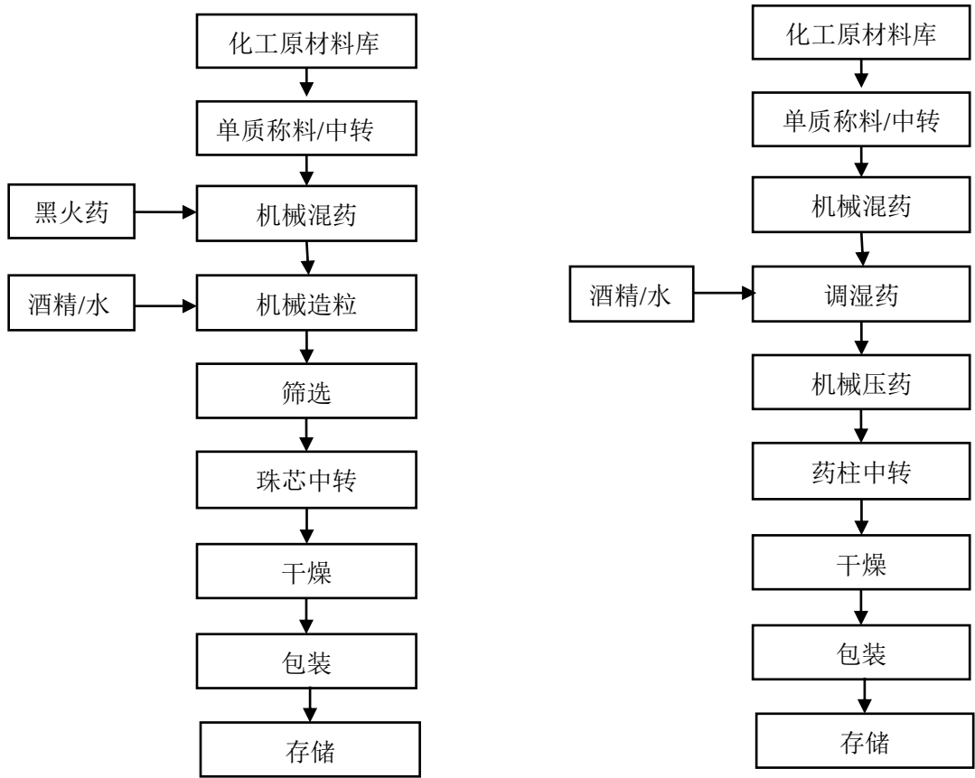
图 2.3.2 -8 烟火药（亮珠、药柱）生产工艺流程图
