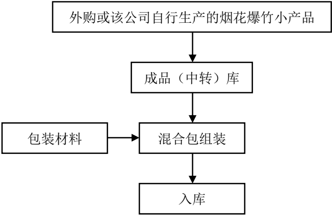
图 2.3.2-7 混合包生产工艺流程图
