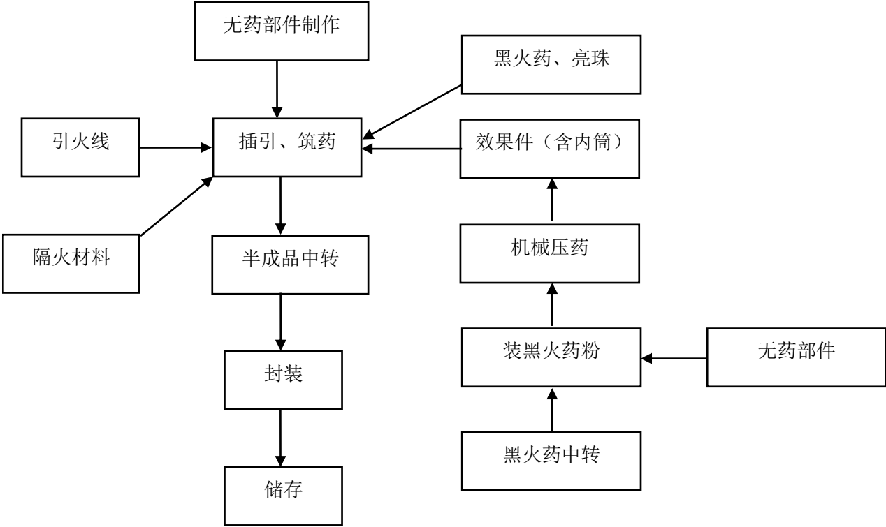
图 2.3.2-3 吐珠类生产工艺流程图
