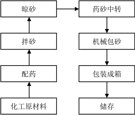
图 2.3.2-6 玩具类（砂炮）生产工艺流程图
