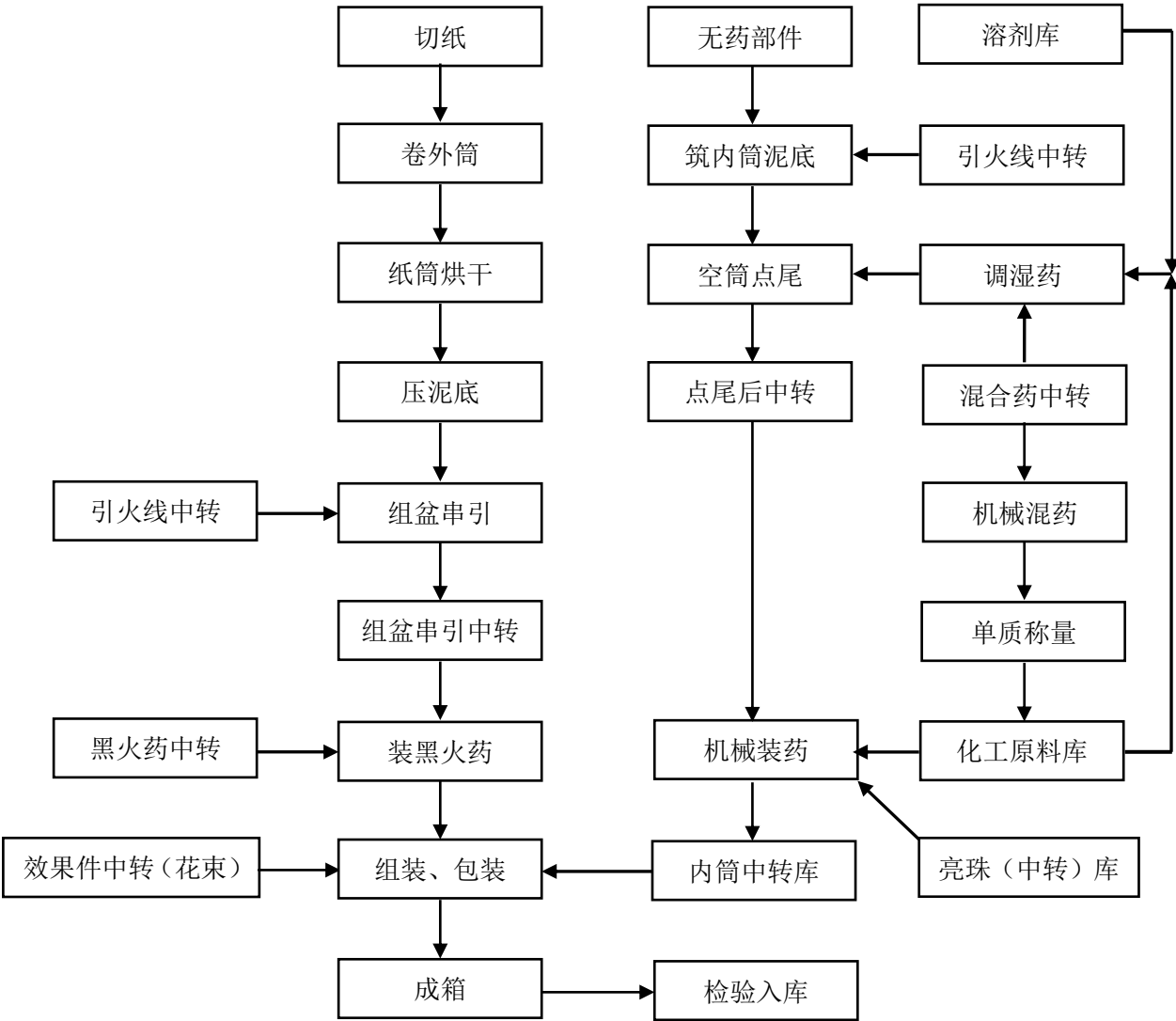
图 2.3.2-2 组合烟花类（机械装药）生产工艺流程图
