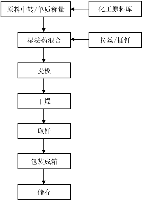
图 2.3.2-4 玩具类（电光花）生产工艺流程图
