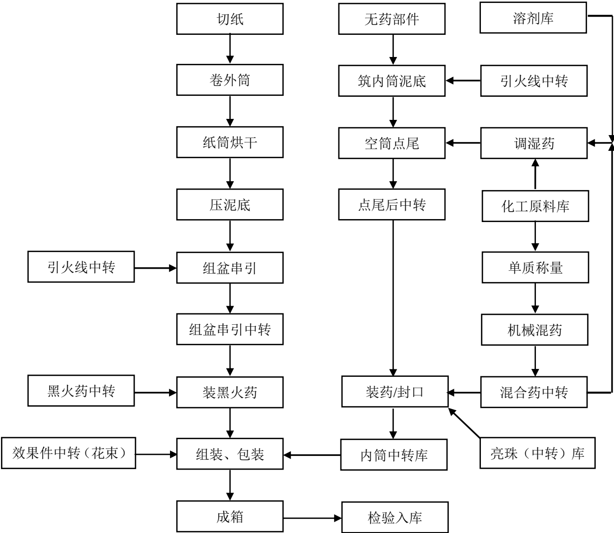
图 2.3.2-1 组合烟花类（手工装药）生产工艺流程图
