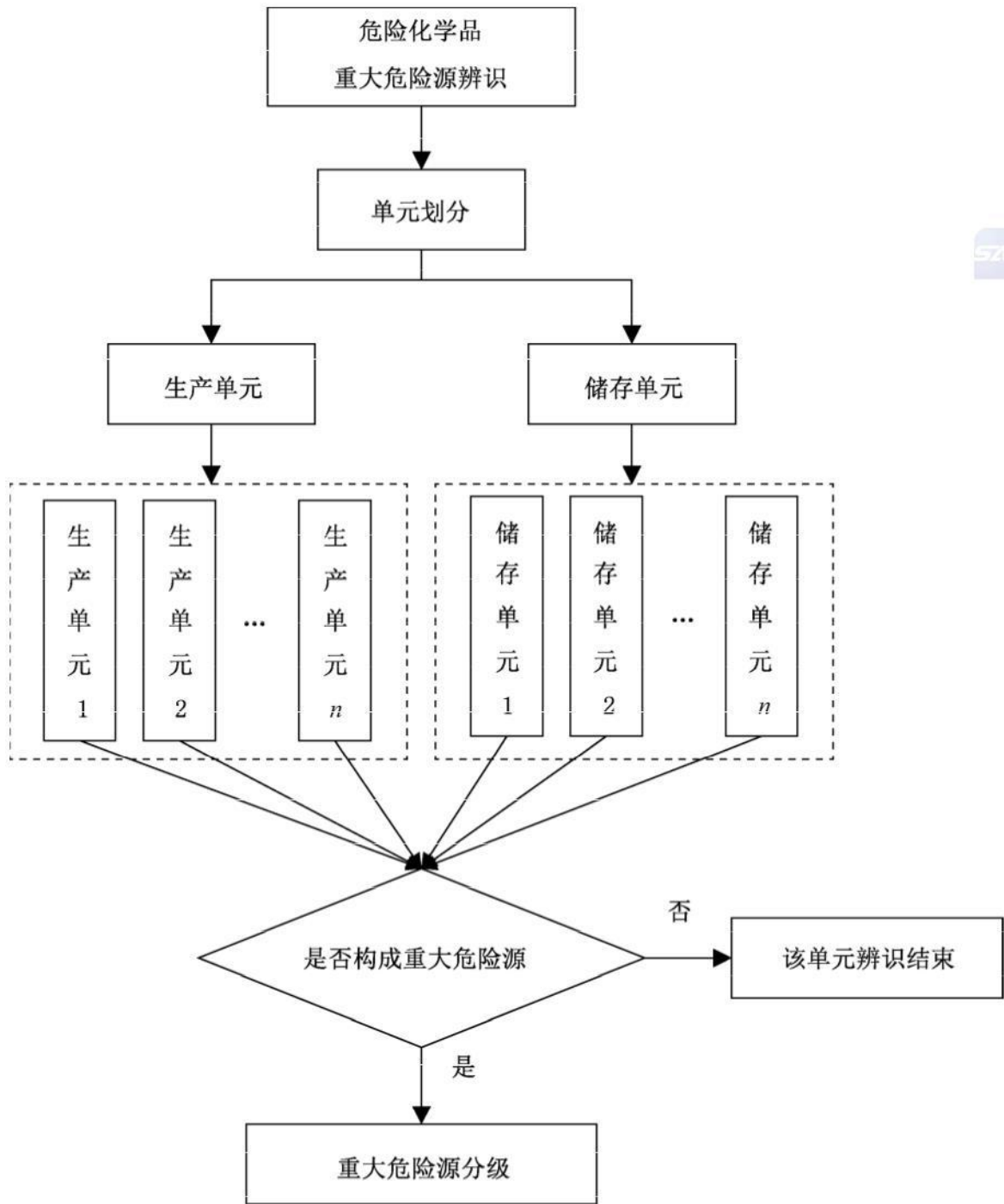
图3.4-1 重大危险源辨识流程表
