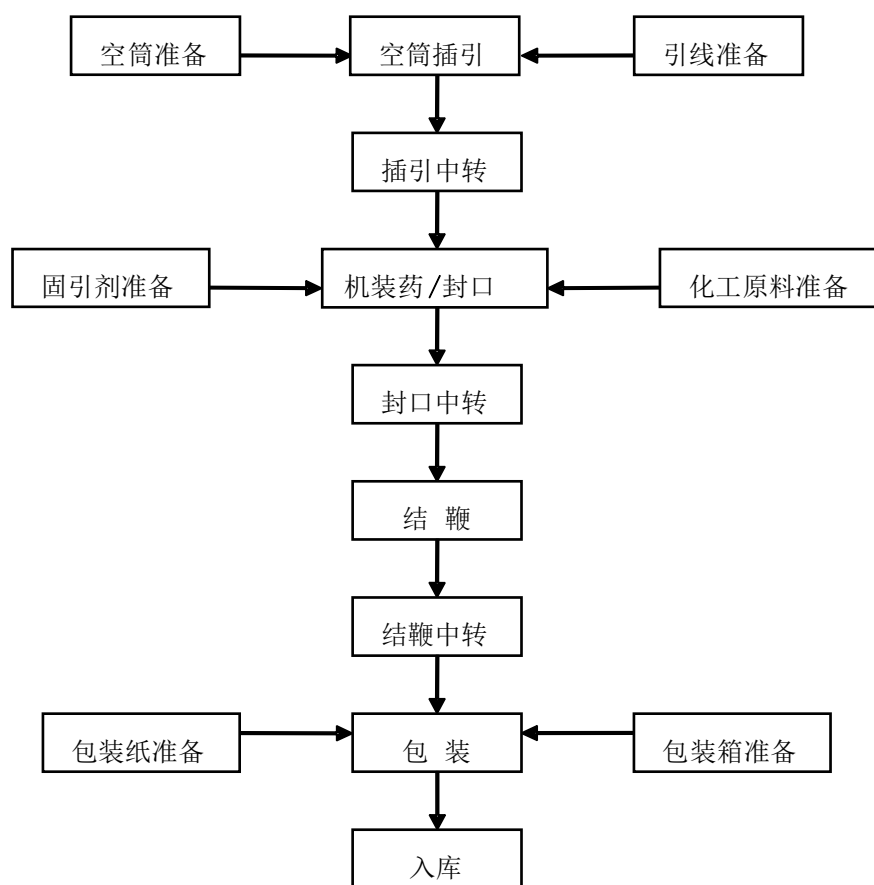
图 2-4-4 爆竹类产品生产工艺流程图
