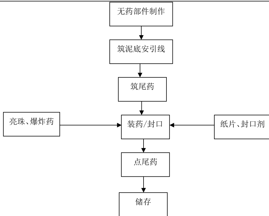
图 2-4-2 效果内筒生产流程
