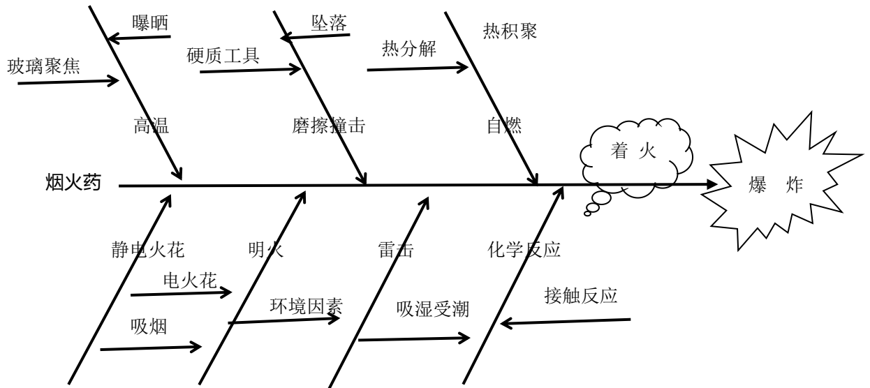
图 3-14-1 烟火药燃烧、爆炸触发条件分析图
