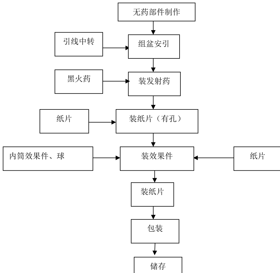
图 2-4-3 组合烟花生产流程图
