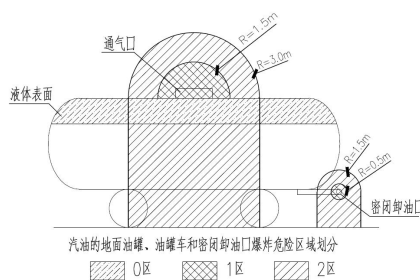
F3.3-2 汽油的油罐车和密闭卸油口的爆炸危险区域划分
