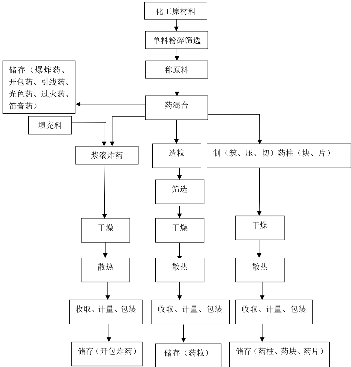
图 2-4-2 药物裸药效果件生产流程图
