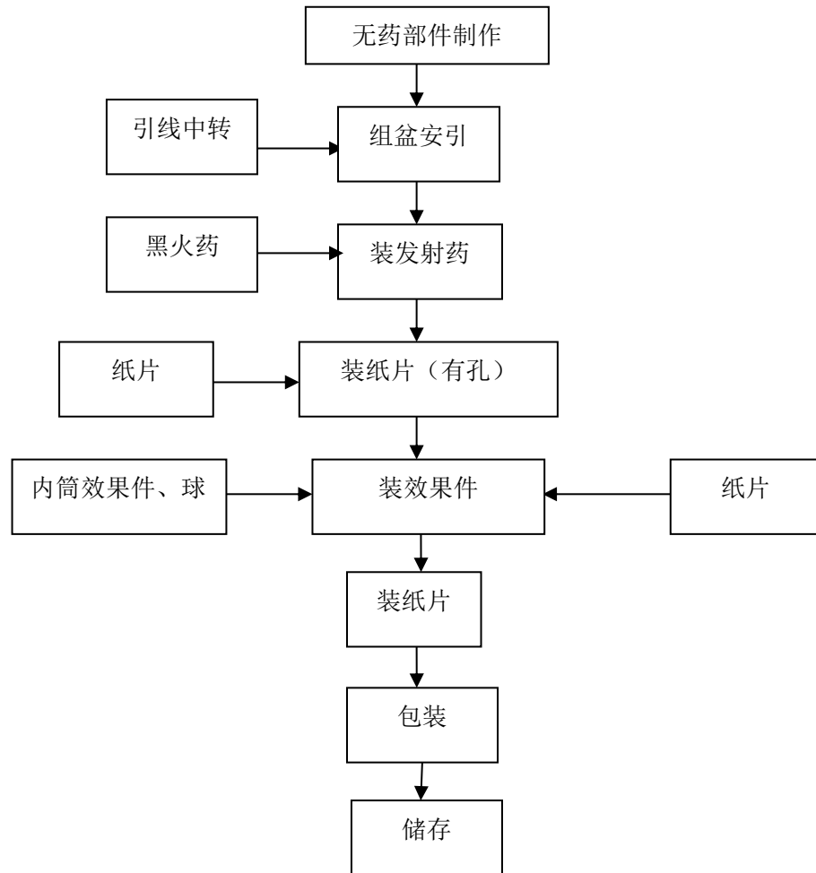
图 2-4-3 组合烟花生产流程图
