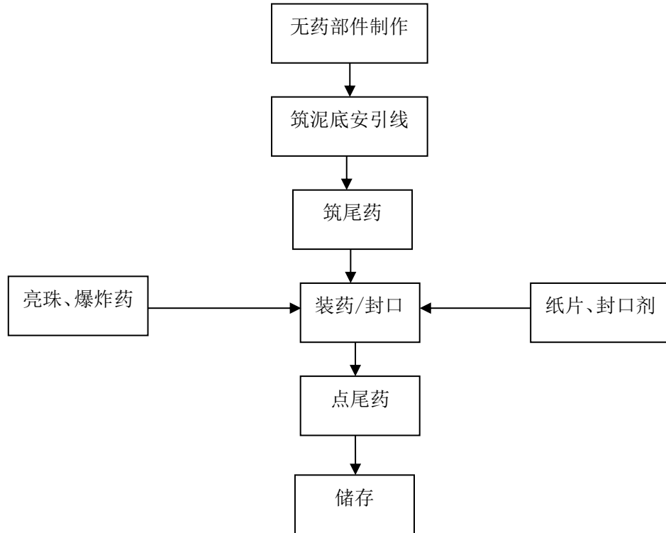
图 2-4-1 效果内筒生产流程
