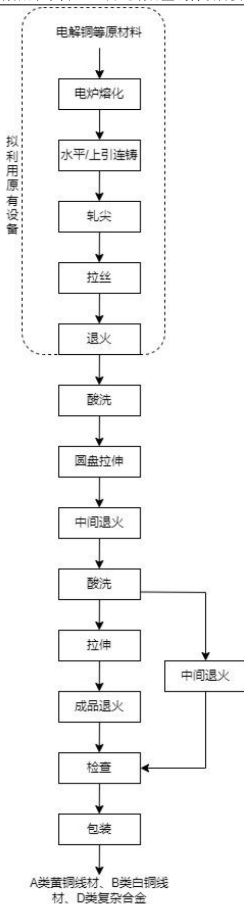
图 2.7-1 连铸制坯法生产工艺流程图
