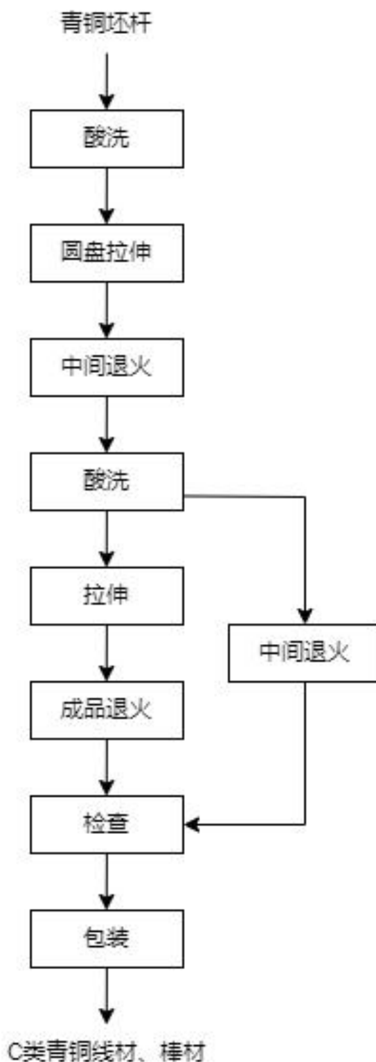
图 2.7-2 孔型轧制生产工艺流程图
