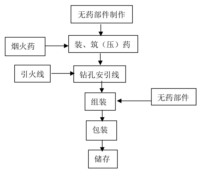
图 2-4-4 旋转升空类（无翅、有翅）生产工艺流程图
