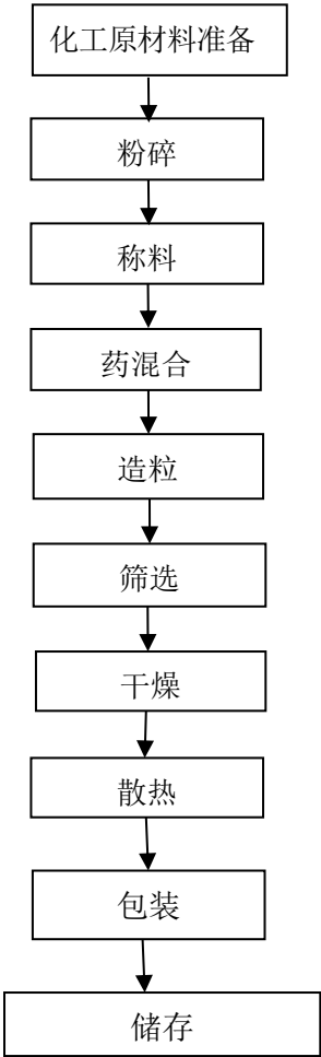
图 2-4-1 药物裸药效果件（亮珠）生产工艺流程图
