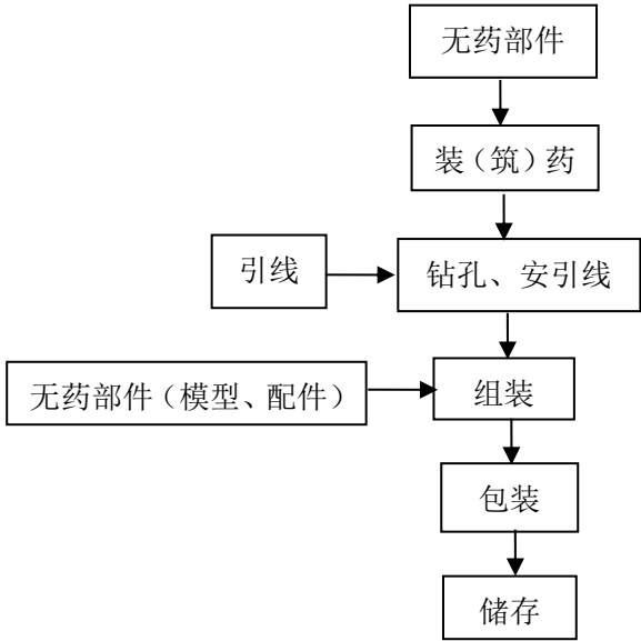
图 2-4-5 造型玩具类生产工艺流程图
