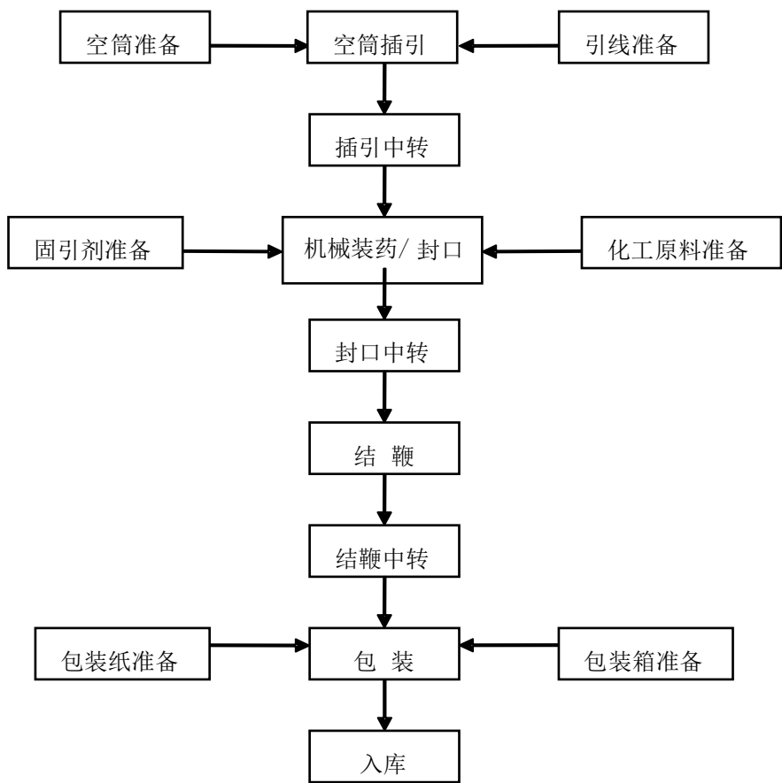
图 2-4-6 爆竹类产品生产工艺流程图
